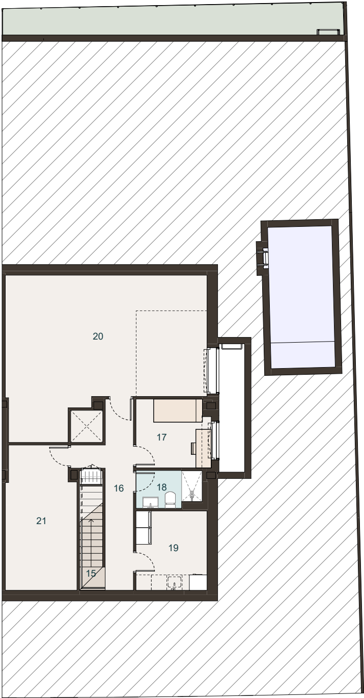
PLANTA SÓTANO
