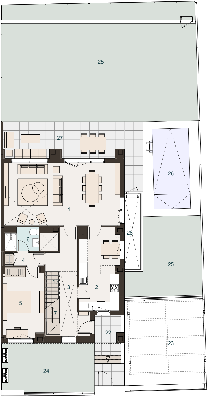
PLANTA BAJA
